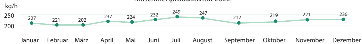
Maschinenproduktivität 2022
